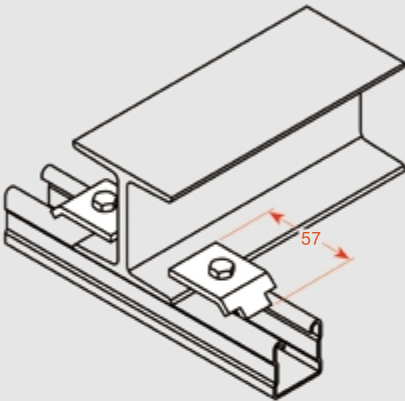
CAP042 Wt 0.10kg 单孔连接梁盖板
