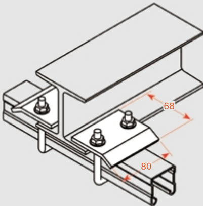
CAP043 Wt 0.31kg U型螺栓固定板
