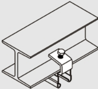
CAP044 Wt 0.13kg 轻载连接梁盖板
