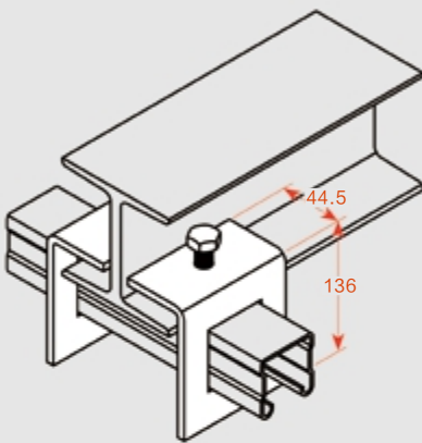
CAP041 Wt 0.35kg 7型支架
